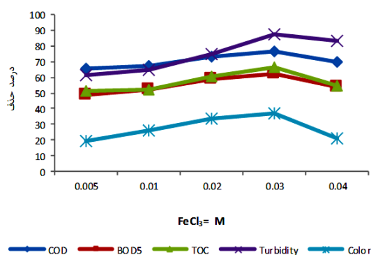
نمودار شماره ۲: نتایج حاصل از تاثیر تغییرات غلظت یون های آهن
