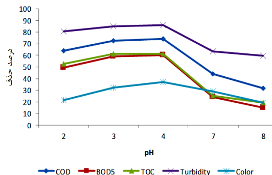
نمودار شماره ۳: نتایج حاصل از تاثیر pH های مختلف بر کارایی فرایند فنتون
