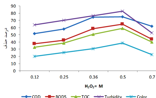
نمودار شماره ۱: نتایج حاصل از تغییرات غلظت هیدروژن پراکسید
