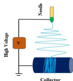
تصویر شماره 1: تصویر شماتیک فرایند الکترورسی
