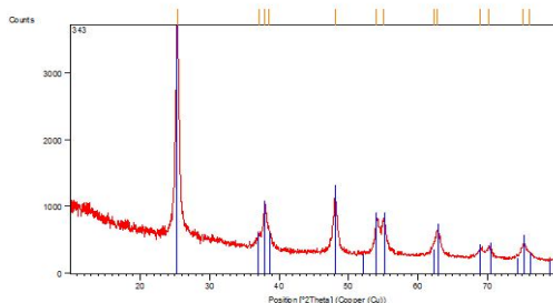
تصویر شماره 3: الگوی XRD نانوذرات تیتانیوم دی اکسید ستر شده با استفاده از یک گرم عصاره خشک و 3/75 میلی لیتر محلول تیتانیوم
