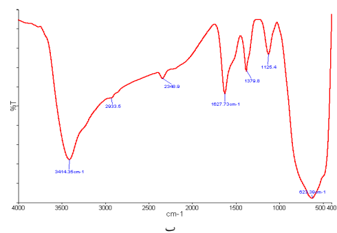
تصویر شماره 4: طیف سنجی FTIR (الف) عصاره برگ حرا و (ب) نانوذرات تیتانیوم دی اکسید نمونه S2 ستر شده با استفاده از عصاره برگ حرا
