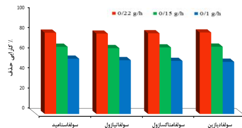
نمودار شماره ۸: اثر غلظت گاز ازن ورودی بر تجزیه آنتی بیوتیک های سولفانامید
