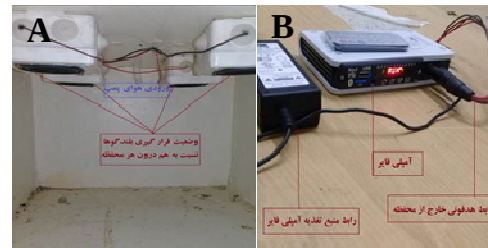
تصویر شماره 1: فضای داخلی محفظه‌های صوتی بازآوا (A) و فضای خارجی آن همراه با آمپلی فایر (B)
