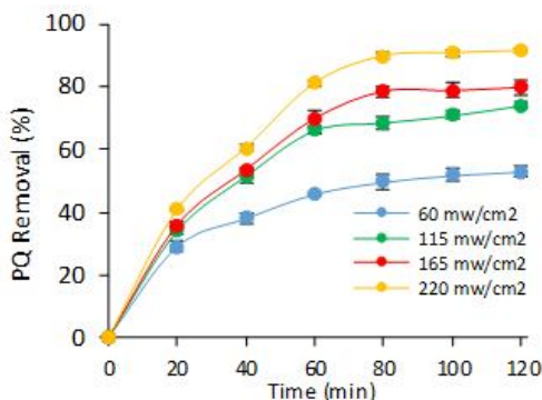
نمودار شماره 4: تاثیر روند تغییرات شدت نور فرابنفش بر تخریب فتوکاتالیستی آفت کش پاراکوات در فرایند ZG/UV (7=pH)، بارگذاری کاتالیست=10 درصد، غلظت کاتالیست=0/5 گرم در لیتر، غلظت آلاینده=10 میلی گرم در لیتر)
