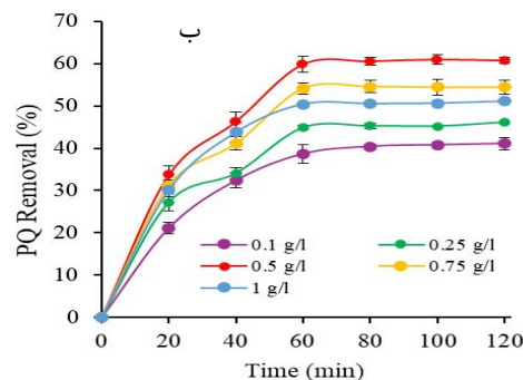
نمودار شماره 3: الف - تاثیر غلظت کاتالیست ZG و ب - تاثیر غلظت پاراکوات بر تخریب آن در فرایند ZG/UV (7 = pH)، بارگذاری کاتالیست=10، غلظت کاتالیست=0/5 گرم در لیتر، غلظت آلاینده=30 میلی گرم در لیتر، شدت نور فرابنفش (115 mw/cm 2 )
