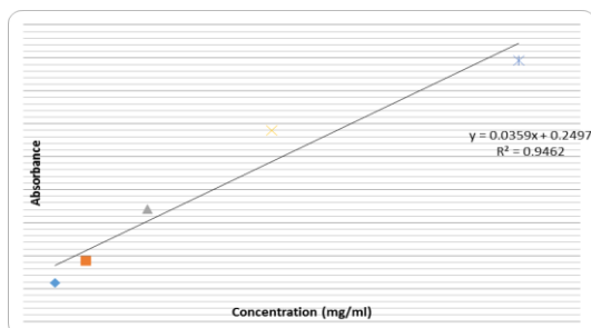
نمودار شماره ۱: منحنی استاندارد ترکیب گالیک اسید
