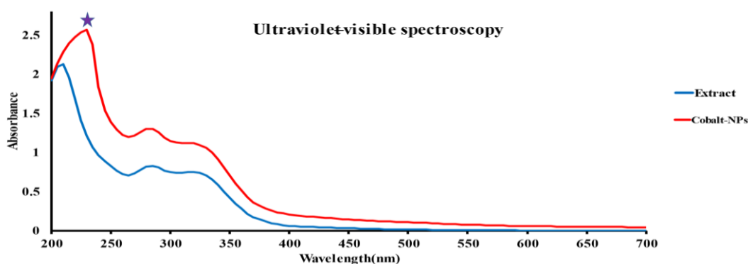
نمودار شماره ۱: طیف سنجی جذبی UV نانوذرات کبالت در مقایسه با عصاره کوتکوتو (★: پیک نشان دهنده تشکیل نانوذرات)
