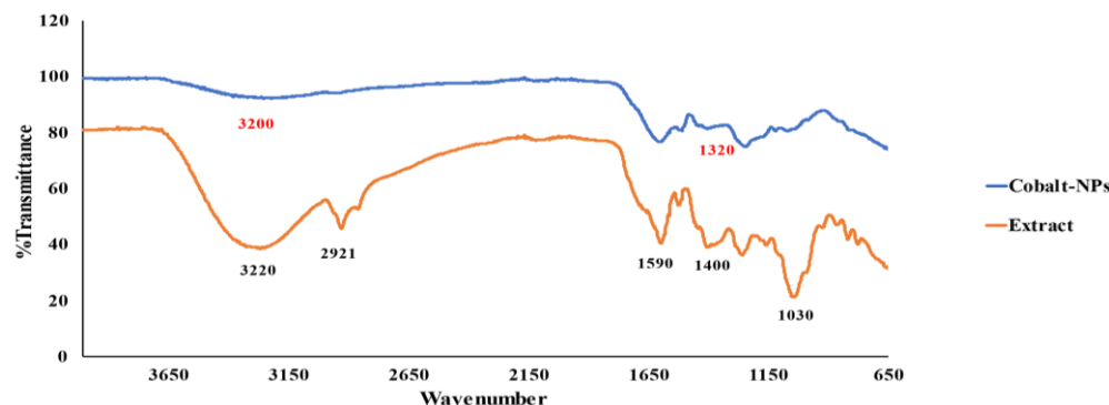
نمودار شماره ۴: طیف FT-IR نانوذرات کبالت سنتز شده با استفاده از عصاره کوکتوتو
