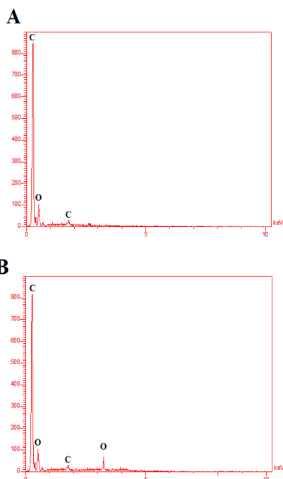
نمودار شماره ۲: طیف سنجی پراش انرژی پرتو ایکس (EDX) داربست نانوفایبری PCL (A) و داربست نانوفایبری PCL حاوی آرت میسینین (B)
