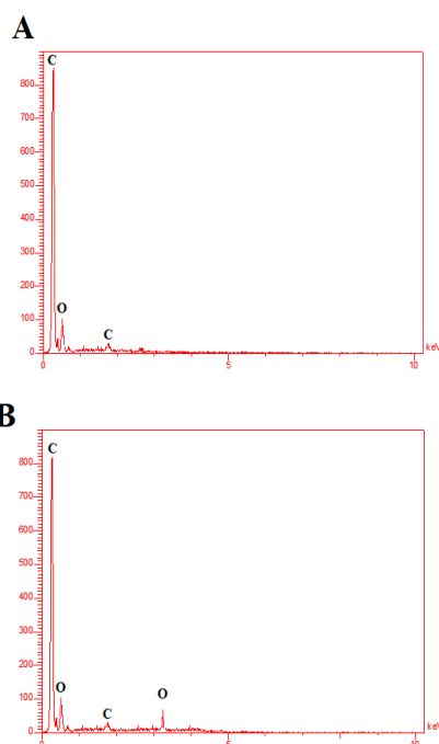
نمودار شماره ۲: طیف سنجی پراش انرژی پرتو ایکس (EDX) داربست نانوفایبری PCL (A) و داربست نانوفایبری PCL حاوی آرتمیسنین (B)
