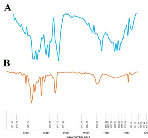
نمودار شماره ۱: طیف FT-IR مربوط به داربست PCL (A) و داربست PCL حاوی Art (B). پیکنهای جذب در 3512 \text{ cm}^{-1} و 3621 \text{ cm}^{-1} مشاهده شده به ترتیب مربوط به گروه هیدروکسیل و ارتعاشات کششی C-O می باشد.
