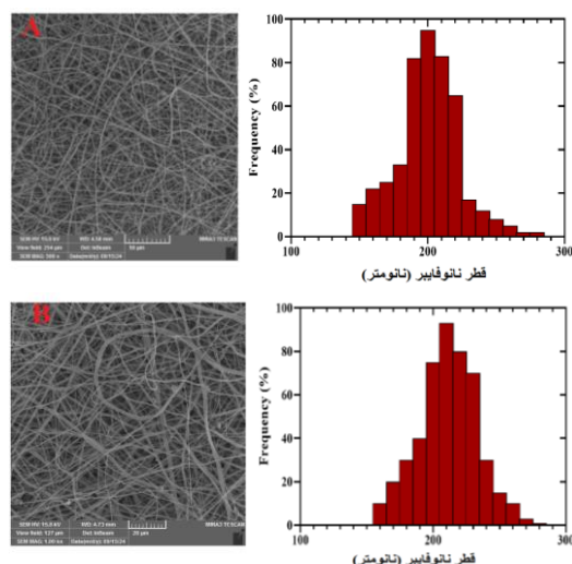
تصویر شماره ۱: (A) داربست PCL، (B) داربست PCL-PEG حاوی Art. می‌توان مشاهده کرد که سطح نانوفایر صاف بوده و هیچ کریستالی از آرتمیسنین روی سطح نانوفایرها دیده نمی‌شود.
