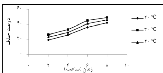
نمودار شماره ۲: تاثیر دما بر میزان جذب فنل بر روی خاکستر پر (زمان: ۲ تا ۸ ساعت؛ pH=۳؛ غلظت فنل: ۱۵ میلی گرم بر لیتر؛ مقدار جاذب ۲ گرم)
