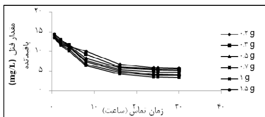
نمودار شماره ۴: تاثیر زمان تماس بر میزان جذب فنل بر روی خاکستر پر (pH=۳؛ دما: ۳۰ درجه؛ غلظت فنل: ۱۵ میلی گرم بر لیتر؛ مقدار جاذب ۰/۲ تا ۲ گرم)
