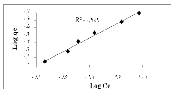
نمودار شماره ۶: ایزوترم خطی جذب فروندلیش برای فتل توسط پر شتر مرغ در دمای ۳۰ °C
