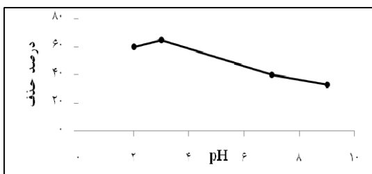
نمودار شماره ۱: تاثیر pH بر میزان جذب فنل بر روی خاکستر پر (زمان: ۸ ساعت؛ دما: ۳۰ درجه؛ غلظت فنل: ۱۵ میلی گرم بر لیتر؛ مقدار جاذب: ۲ گرم)
