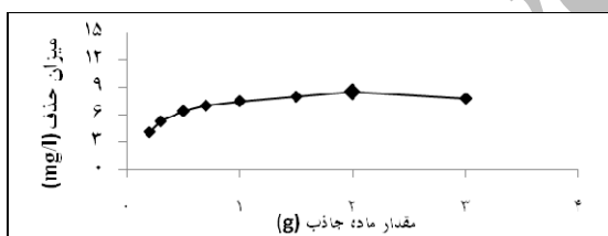
نمودار شماره ۳: تاثیر مقدار ماده جاذب بر میزان جذب فنل بر روی خاکستر پر (زمان: ۸ ساعت؛ pH=۳؛ دما: ۳۰ درجه؛ غلظت فنل: ۱۵ میلی گرم بر لیتر)
