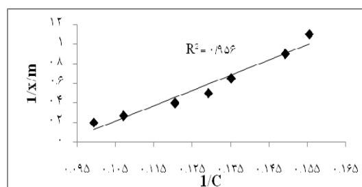
نمودار شماره ۷: ایزوترم خطی جذب لانگمیر برای فتل توسط پر شتر مرغ در دمای ۳۰ °C
