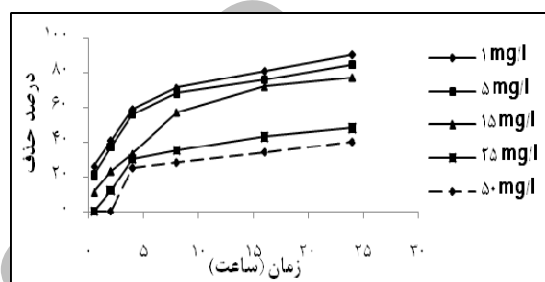
نمودار شماره ۵: تأثیر غلظت اولیه فتل بر میزان جذب بر روی خاکستر پرشتر مرغ در شرایط بهینه (pH=۳، دما: ۳۰ درجه؛ مقدار جاذب: ۲ گرم؛ زمان از ۰/۵ تا ۲۴ ساعت)
