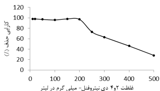
نمودار شماره ۴: تاثیر غلظت اولیه ۴و۲ دی نیترو فلن بر کارایی جذب (pH 5، دوز جاذب ۰/۴ گرم در لیتر و زمان تماس ۱۰۰ دقیقه)
