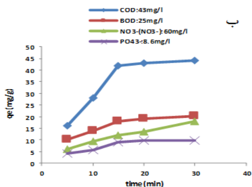
نمودار شماره ۲: تاثیر زمان تماس (الف) بر فرآیند جذب PO 4 3- , NO 3 - , BOD 5 , COD و (ب) ظرفیت جذب با MNPs Fe 3 O 4 (مقدار جاذب به ترتیب ۰/۵ g/l، زمان: متغیر، pH=۵)
