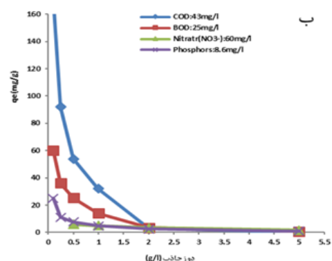
نمودار شماره ۴: تاثیر دوز جاذب بر (الف) فرآیند جذب \text{PO}_4^{3-} , \text{NO}_3^- , COD, BOD 5 و (ب) ظرفیت جذب با MNPs \text{Fe}_3\text{O}_4 (مقدار جاذب: متغیر، زمان: ۱۵min، pH=۳)
