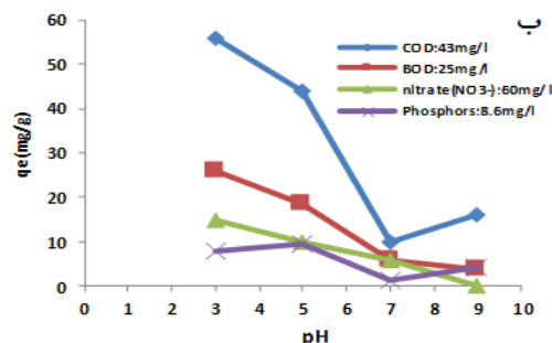
نمودار شماره ۳: تاثیر pH بر (الف) فرآیند جذب PO 4 3- , NO 3 - , BOD 5 , COD و (ب) ظرفیت جذب با MNPs Fe 3 O 4 (مقدار جاذب: ۰/۵ g/l، زمان: ۱۵ min، متغیر: pH)
