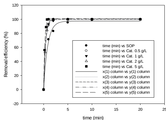
نمودار شماره ۱: مقایسه راندمان های حذف کلیفرم در غلظت های مختلف کاتالیست با جمعیت اولیه میکروبی ml MPN/100 ۳/۲×۱۰
