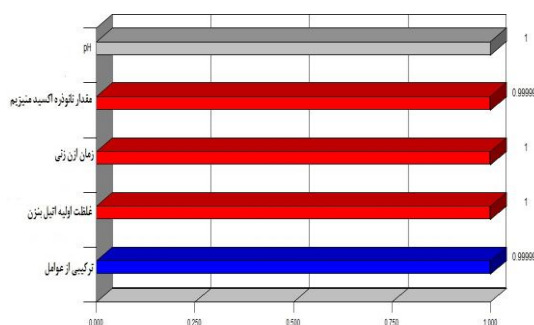
تصویر شماره ۵: الف. شرایط بهینه طراحی شده با روش سطح پاسخ جهت حذف اتیل بنزن توسط فرآیند ازن زنی کاتالستی با استفاده از نانو ذرات اکسید منیزیم. ب. نمودار میله ای ضرایب تمایل هر یک از متغیرها در شرایط بهینه
