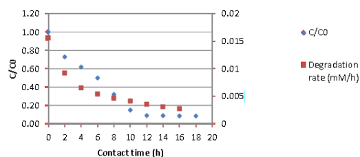
نمودار شماره ۴: غلظت باقیمانده و نرخ تجزیه آلایندہ ۴و۲-دی نیتروفل در مقادیر مختلف زمان ماند، 2,4-DNP=۱۰ ppm؛ ABTS=۱ mM؛ pH=۵؛ دما=۵۰ °C
