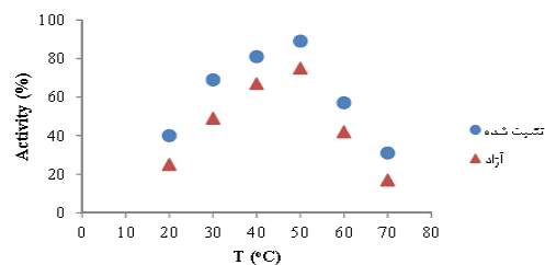
نمودار شماره ۳: مقایسه تاثیر متغیر دما بر عملکرد آنزیم لکاز آزاد و تثبیت شده، ABTS=۱ mM؛ pH=۵
