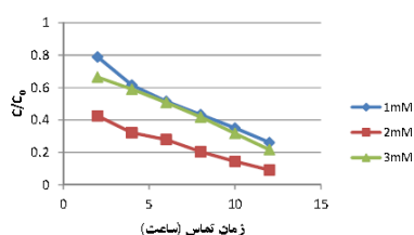
نمودار شماره ۷: تاثیر غلظت مدیاتور بر تجزیه آلاینده ۴،۲-دی نیتروفنل توسط سیستم آنزیمی لکاز تثبیت شده، pH=۵، 2,4-DNP = ۱۰ ppm، دما=۵۰ °C
