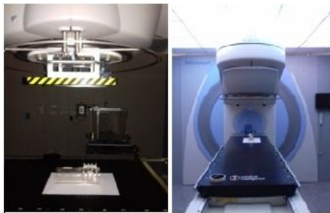
تصویر شماره 3: تابش دهی گروه های درمانی با فیکس کردن حیوانات در میدان 10 \times 10 شتاب دهنده خطی 6MV Elekta Compact
