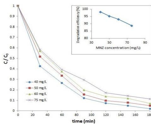
نمودار شماره ۳: تأثیر غلظت اولیه مترونیدازول بر راندمان حذف (pH ۸، دوز کاتالیست ۱/۵ g/L)
