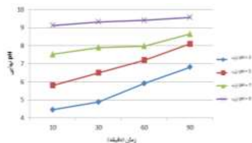
تصویر شماره ۷: تغییرات pH اولیه پسب در اختلاف پتانسیل ۶ ولت در زمان های مختلف
