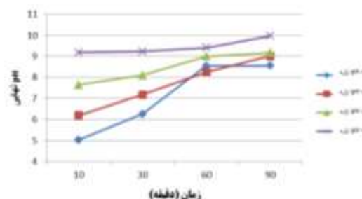
تصویر شماره ۸: تغییرات pH اولیه پسب در اختلاف پتانسیل ۱۲ ولت در زمان های مختلف
