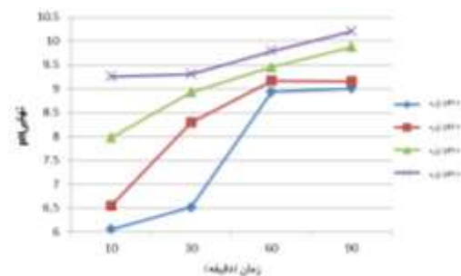
تصویر شماره ۹: تغییرات pH اولیه پسب در اختلاف پتانسیل ۱۸ ولت در زمان های مختلف
