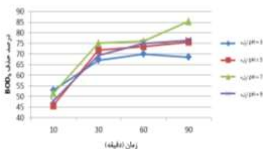
تصویر شماره ۷: درصد حذف COD در اختلاف پتانسیل ۶ ولت در pH و زمان های مختلف
