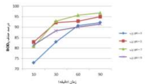
تصویر شماره ۹: درصد حذف BOD5 در اختلاف پتانسیل ۱۸ ولت در pH و زمان های مختلف
