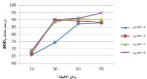
تصویر شماره ۸: درصد حذف BOD5 در اختلاف پتانسیل ۱۲ ولت در pH و زمان های مختلف
