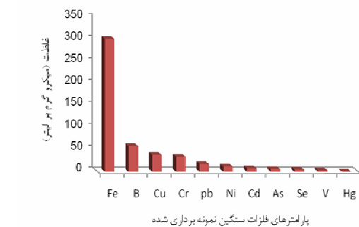
شکل شماره ۱: نمودار میانگین غلظت فلزات سنگین در چاه نیمه‌ها
