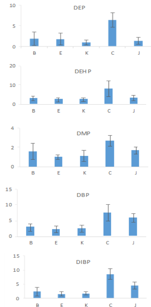
نمودار شماره ۵: نمودارهای میانگین غلظت استرهای فتالات برحسب ppb در آب‌های بطری شده تحت شرایط محیطی بعد از ۵ روز (B) = دمای انجماد (-۱۸°C)، E = دمای یخچال (۴°C)، K = دمای انکوباتور (۲۵°C)، C = دمای انکوباتور (۴۲°C)، J = نور خورشید (۲۳±۲°C)
