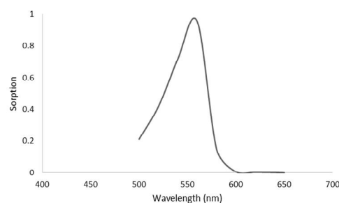
تصویر شماره 6: طیف جذبی رودامین B با غلظت اولیه 1 mg/L
