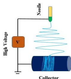
تصویر شماره 1: تصویر شماتیک فرایند الکتروریسی
