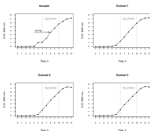
تصویر شماره 3: منحنی رشد سویه نیا (Ancestor) و سویه های تکامل یافته (Evolved 1-3)
