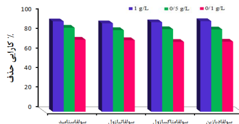
نمودار شماره ۷: اثر غلظت کاتالیز بر تجزیه آنتی بیوتیک های سولفانامید
