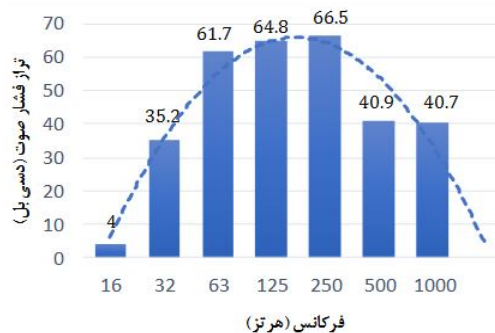
تصویر شماره 1: آنالیز فرکانس صدای کم فرکانس (در یک اکتافاوند) توسط صداسنج با شبکه وزنی A (Casella CEL-450)
