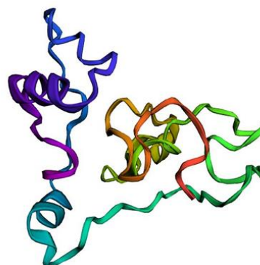
تصویر شماره ۳: تصویر از مدل سه بعدی ساخته شده برای پروتئین طراحی شده توسط نرم افزار آنالیز SAVES v6.0. سمت چپ آبی رنگ انتهای N و سمت راست تصویر سبز رنگ انتهای C می باشد.
