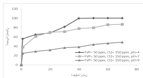
نمودار شماره ۳: بررسی تأثیر pH مختلف بر حذف فاویپیراویل در واکنش با کلر
