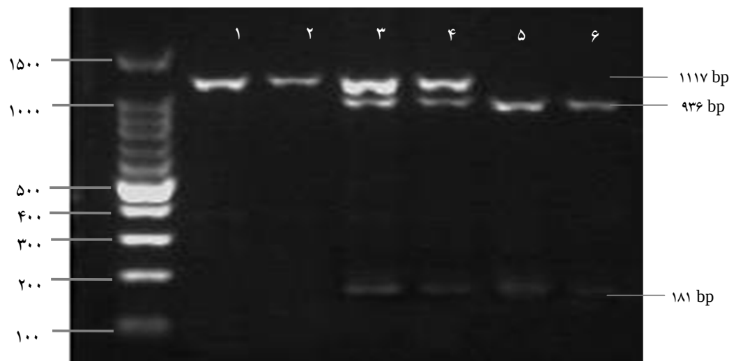
تصویر شماره ۱: محصولات RFLP برای ژن HSP70-2 بر روی ژل آگارز ۲ درصد. باند ۱۱۱۷ bp در نمونه‌های ۱ و ۲ بیانگر ژنوتیپ AA، سه باند ۱۱۱۷، ۹۳۶، ۱۸۱ bp در نمونه‌های ۳ و ۴ نشانگر ژنوتیپ AG و دو باند ۱۸۱ و ۹۳۶ bp در نمونه‌های ۵ و ۶ نمایانگر ژنوتیپ GG می‌باشد. ردیف M مربوط به نشانگر ۱۰۰ bp
