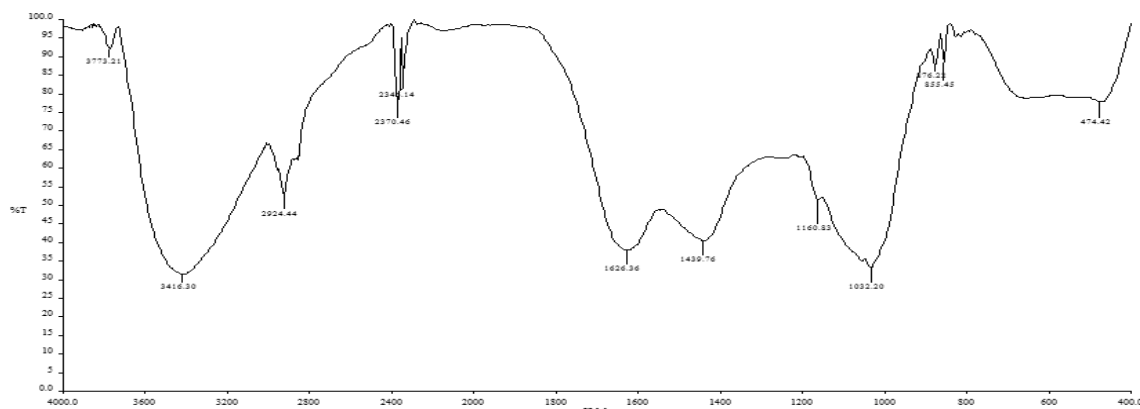
نمودار شماره ۱: طیف اسپکتروفتومتری مادون قرمز تبدیل فوریه مربوط به جلبک Padina sanctae cruces
