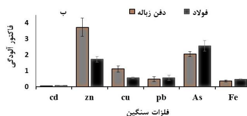
تصویر شماره ۱: میانگین شاخص زمین‌انباشتگی (الف) و فاکتور آلودگی (ب) فلزات سنگین در مناطق مورد مطالعه. میله‌ها نشان دهنده خطای استاندارد است.
