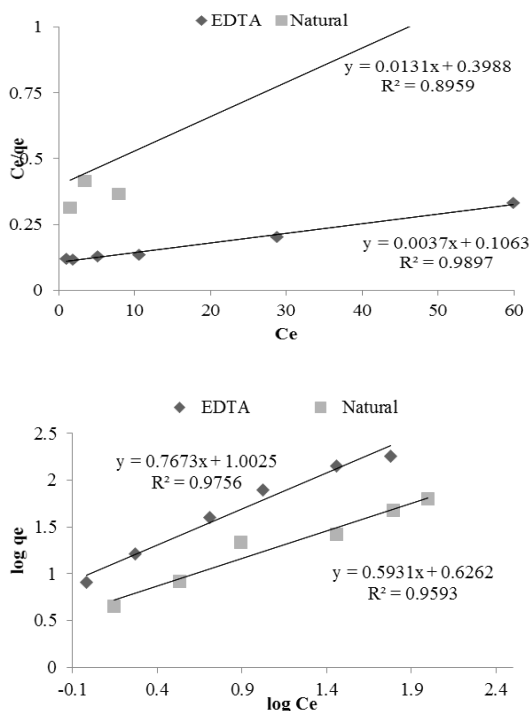
نمودار شماره ۶: مدل ایزوترم لانگمویر (a) و فروندلیچ (b) برای نانورس خام و اصلاح شده با EDTA
