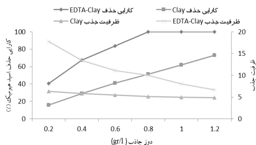
نمودار شماره ۴: تأثیر دوز جاذب برای نانورس اصلاح شده با EDTA و نانورس خام در pH=۲ و غلظت اسید ۸ mg/l هیومیک
