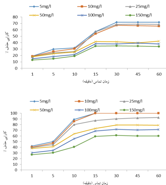
نمودار شماره ۵: نمودار غلظت- زمان برای نانورس خام (الف) و نانورس اصلاح شده با EDTA (ب) در pH=2
