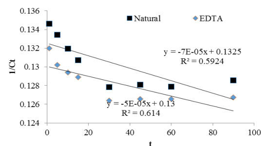
نمودار شماره ۲: مدل سینتیک درجه اول کاذب (a) و درجه دوم کاذب (b) برای نانورس خام و اصلاح شده با EDTA
