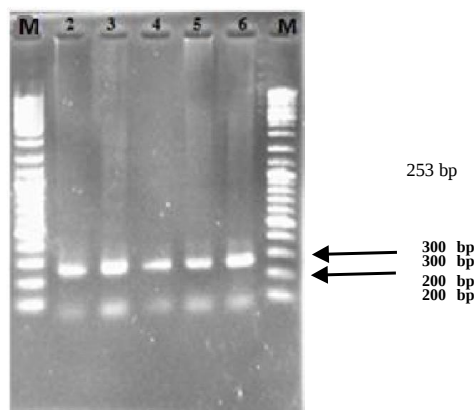
تصویر شماره ۱: الکتروفورز محصولات حاصل از تکثیر قطعه ۲۵۳ جفت بازی پروموتور P2 ژن bcl2 در ژل آگاروز ۱/۵ درصد (چاهک های ۲، ۳، ۴، ۵ و ۶: قطعه ۲۵۳ جفت بازی تکثیر شده در تعدادی از نمونه های بیمار. چاهک M مارکر ۱۰۰ جفت بازی شرکت فرمنتاس)
