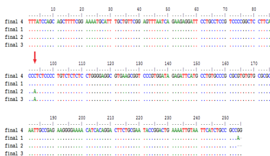
تصویر شماره ۲: هم ردیفی چندتایی (Multiple Alignment) توالی نوکلئوتیدی قطعه ۲۵۳ جفت بازی پروموتور P2 ژن bcl2 با روش ClustalW (فلش نشان دهنده جایگاه A>C۹۳۸- پروموتور P2 ژن bcl2 است که دارای چند شکلی می باشد. نقاط، نشان دهنده حضور نوکلئوتید یکسان در محل مورد نظر است.)
