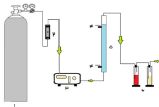
تصویر شماره ۱: مشخصات راکتور مورد استفاده در این تحقیق (۱) - منبع اکسیژن ۲ - فلومتر ۳ - ازن ژنراتور ۴ - شیر نمونه‌برداری ۵ - راکتور تماس ۶ - گازشوی های حاوی محلول یدید پتاسیم
