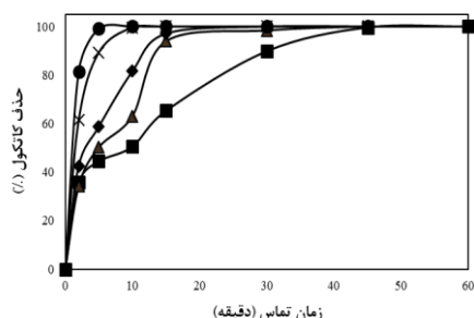
نمودار شماره ۴: تأثیر غلظت اولیه کاتکول بر راندمان حذف آن در فرایند COP (غلظت کاتکول ۱۰۰۰ mg/l، pH=۸، دوز کاتالیست ۳ gr/L و دوز ازن ۰/۳۸ gr/hr)
