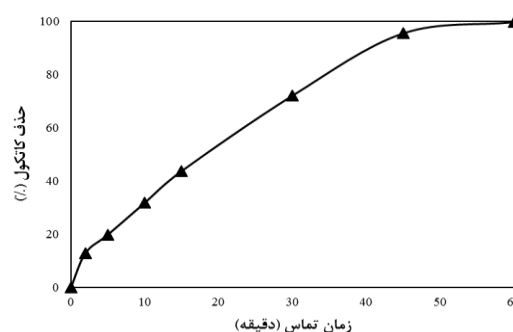
نمودار شماره ۲: تأثیر زمان واکنش بر راندمان حذف کاتکول در فرایند COP (غلظت کاتکول ۱۰۰۰ mg/l، pH=۸، دوز کاتالیست ۰/۳۸ gr/L و دوز ازن ۰/۳۸ gr/hr)
