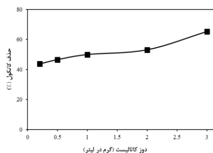
نمودار شماره ۳: تأثیر دوز اولیه کاتالیست بر راندمان حذف کاتکول در فرایند COP (غلظت کاتکول ۱۰۰۰ mg/l، pH=۸، دوز ازن ۰/۳۸ gr/hr)
