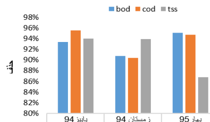
نمودار شماره ۱: کارایی حذف BOD 5 ، COD و TSS در تصفیه خانه فاضلاب ناحیه صنعتی الوند قزوین
