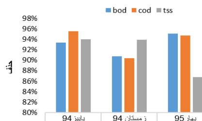
نمودار شماره ۱: کارایی حذف BOD 5 ، COD و TSS در تصفیه خانه فاضلاب ناحیه صنعتی الوند قزوین
