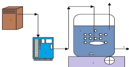
تصویر شماره ۱: شماتیک راکتور مورد استفاده در تحقیق (۱) دستگاه اکسیژن ساز، ۲ دستگاه ازن ساز، ۳ گاز شوی، ۴ میکسر، ۵ شیر نمونه بردار
