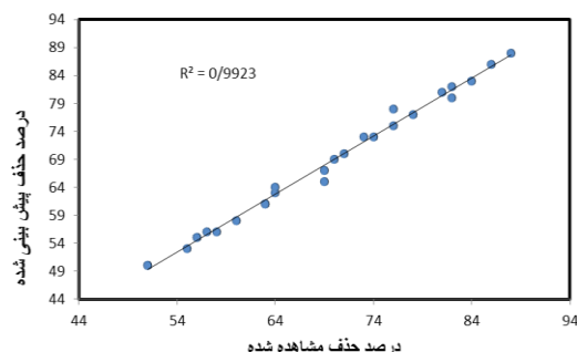
نمودار شماره ۲: نمودار پیش‌بینی شده در مقابل مشاهدات در حذف رنگ از فاضلاب نساجی
