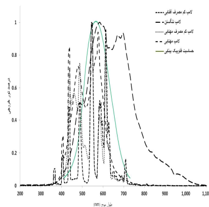
نمودار شماره 2: مقایسه طیف لامپ ها با نمودار حساسیت فتوپیک بینایی انسان.
