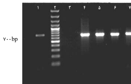
تصویر شماره ۱: چاهک ۱: سویه کنترل مثبت، چاهک M: مارکر ۱۰۰ bp Plus، چاهک ۳: چاهک کنترل منفی، ستون‌های ۴-۶-۷: جدایه‌های بالینی جدا شده از ادرار دارای ژن ant(2'')-Ia ، اندازه محصول PCR، ۷۰۰ bp
