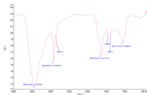
نمودار شماره ۱: تصویر FTIR گیاه آبزی آزولا فلیکولوئیدس به صورت پودر خشک شده قبل استفاده (الف) - بعد از استفاده (ب)
