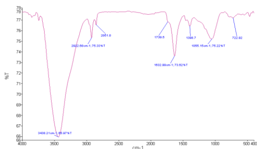
نمودار شماره ۳: تصویر FTIR گیاه آبزی آزولا فلیکولوئیدس به صورت کربن اصلاح شده قبل استفاده (الف) - بعد از استفاده (ب)
