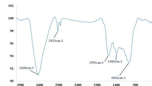
نمودار شماره ۲: تصویر FTIR گیاه آبزی آزولا فلیکولوئیدس به صورت پودر اصلاح شده قبل استفاده (الف) - بعد از استفاده (ب)
