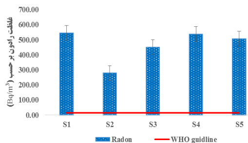
نمودار شماره ۳: میانگین غلظت گاز رادون با در ایستگاه های نمونه برداری
