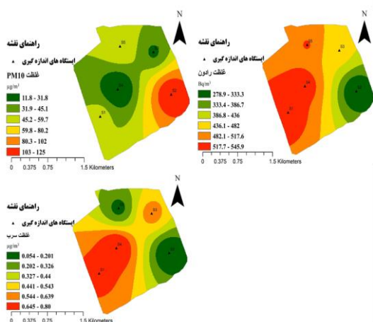
تصویر شماره ۲: پهنه بندی میانگین غلظت PM 10 ، سرب و گاز رادون در ایستگاه های نمونه برداری
