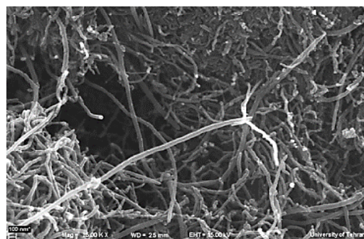
تصویر شماره ۱: میکروسکوپ الکترونی روبشی (SEM) برای نانو تیوب کربنی بهینه شده با Fe_3O_4
