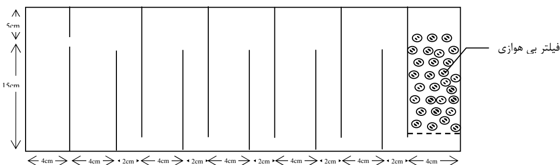
تصویر شماره ۲: طرح شماتیک راکتور ABR-AFR ساخته شده برای تحقیق
