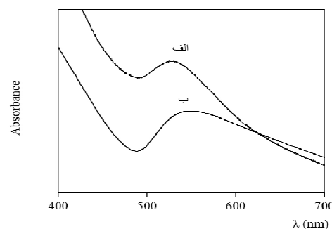
نمودار شماره 1: الف: اسپکتروسکوپی UV-Vis نانوذرات طلا در حضور آپوفریتین، ب: بدون حضور آپوفریتین
