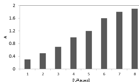
نمودار شماره 5: منحنی اندازه گیری باکتری ویبریوکلرا توسط نانوذره طلای متصل به آنتی بادی OMPW
