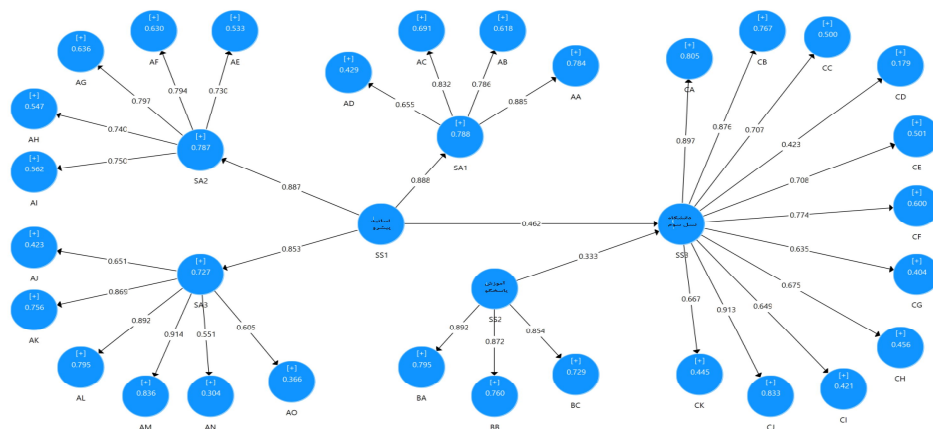
نمودار شماره 1: مدل ساختاری در حالت تخمین استاندارد ضرایب مسیر
