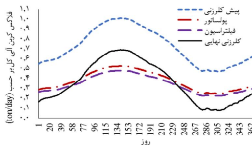
نمودار شماره 3: شبیه سازی تغییرات غلظت و فلاکس کربن آلی کل در واحد های مختلف تصفیه خانه آب تهران پارس
