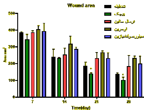
نمودار شماره 1: میانگین مساحت زخم ناشی از سوختگی در گروه های نرمال سالین، اوسرین، سیلورسولفادیازین، پیچک صحرایی و شنبلیله
