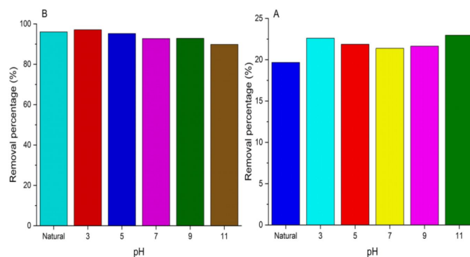
تصویر شماره 3: بررسی اثر pH بر روی کارایی فرآیند جذب AR-18 (A): نانو ذرات MgO و B: PAC؛ شرایط آزمایش: غلظت اولیه AR-18 برابر با 100 mg/L، مقدار ماده جاذب 1 g/L، زمان تماس دو ساعت و دمای 20 °C.
