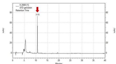
تصویر شماره ۱: آنالیز HPLC برای استاندارد ژینستین با غلظت ۱۲۵ ppm، در آنالیز HPLC انجام شده برای ژینستین با غلظت ۱۲۵ ppm. پیک استاندارد ژینستین در زمان بازداری ۱۰٫۸۱ دقیقه مشاهده می شود.
