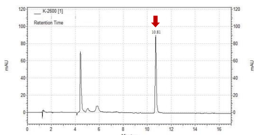
تصویر شماره ۳: تجزیه و تحلیل HPLC برای مخلوط استاندارد ژینستین با عصاره، در نمودار HPLC که از ترکیب استاندارد ژینستین و عصاره تهیه شده است زمان بازداری ۱۰٫۸۱ دقیقه مربوط به پیک ژینستین می باشد.
