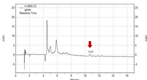
تصویر شماره ۲: دیگرام HPLC عصاره با غلظت ۱۰۰ ppm فلش قرمز رنگ محل پیک ژینستین را در عصاره مشخص می کند.
