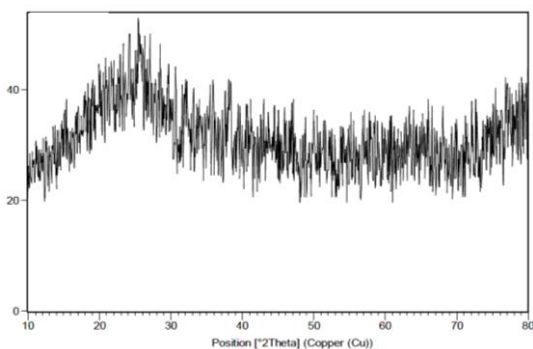
نمودار شماره ۲: الگوی XRD نانوذرات کبالت سنتز شده با استفاده از عصاره گیاهی کوتکوتو
